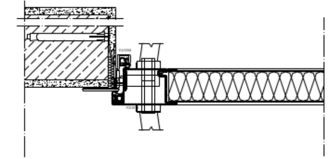
ościeżnica kątowa z uszczelką
