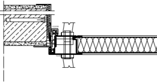
ościeżnica kątowa obejmująca
